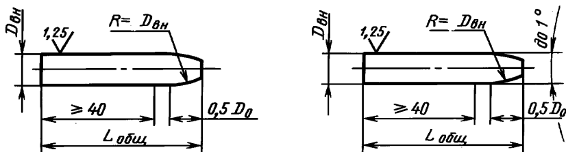
Цилиндрическая пробка
